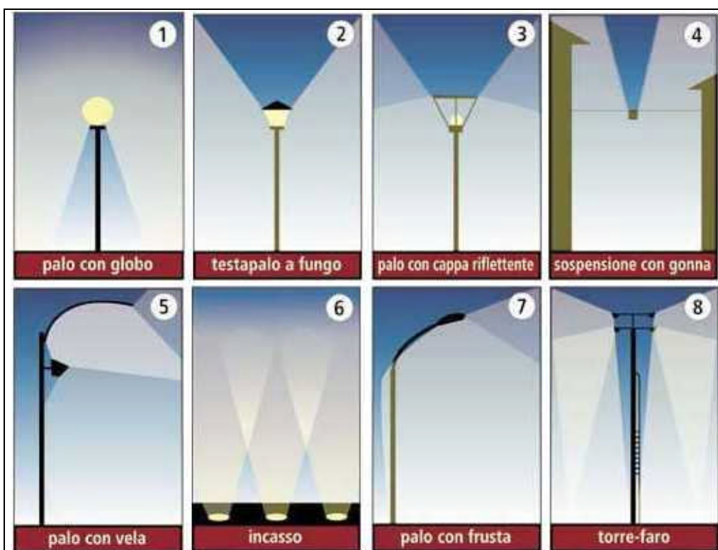
Fig 7 – Impianti di illuminazione NON consentiti dalla D.G.R. 48/31.
