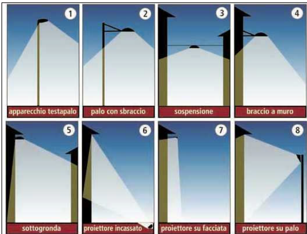
Fig.6 – Impianti di illuminazione conformi alla D.G.R. 48/31. I corpi di cui al punto 6 ed 8 sono ammessi esclusivamente per manufatti di particolare e comprovato valore storico ove non sia possibile illuminarli dall'alto verso il basso.
