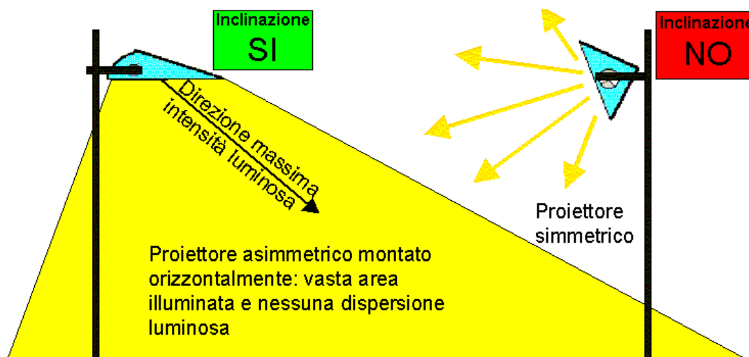
Fig.9 - Apparecchi simmetrici ed asimmetrici se posti con vetro piano orizzontale sono ugualmente conformi alla D.G.R. n. 48/31. In generale tutti i proiettori devono essere installati orizzontali.
