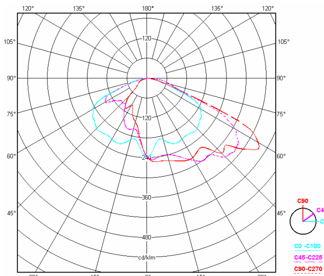
Fig. 6 - Curva fotometrica di apparecchio asimmetrico misurata su 3 piani.
